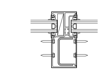
13 STOREFRONT FF451 @ STILE 3" = 1'-0"
